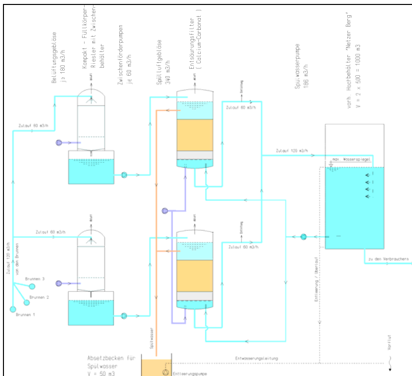
Systemplan
